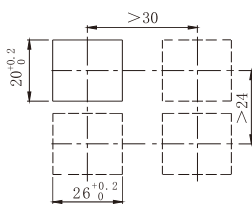
安装长方形平装附件Z14的开孔
