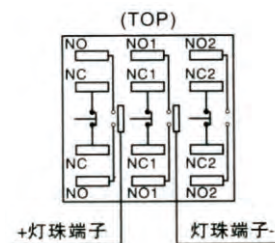
端子排列
