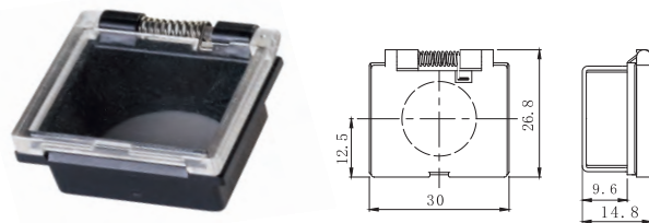
10.长方形平装安全盖AQG16-D
