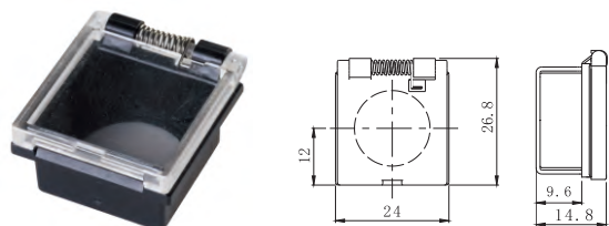
9.方形平装安全盖AQG16-C
