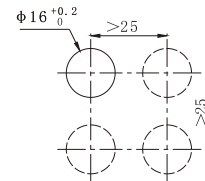
蘑菇形头部的开孔
