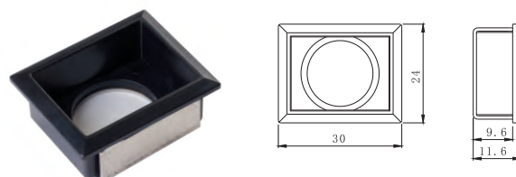
10.长方形平装安全盖AQG16-D
