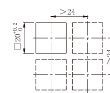
安装方形平装附件Z12的开孔
