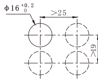
矩形头部的开孔
