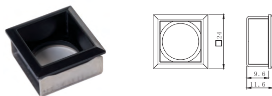
9.方形平装安全盖AQG16-C
