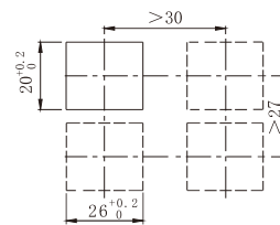
安装平装安全罩AQG16-D的开孔
