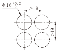
圆形/方形头部的开孔
