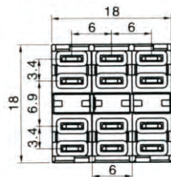
底部视图
